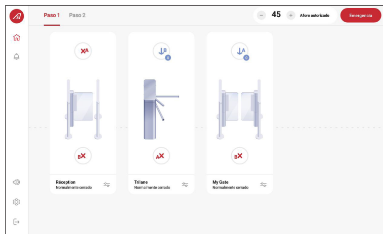
Contador en la pantalla de "Vista de la Batería"
